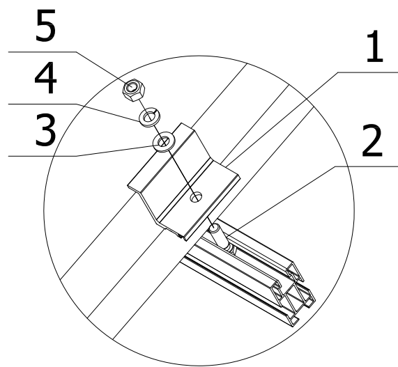
Detalle presor lateral
