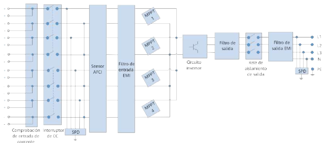
Figura 2-5 Diagrama esquemático
