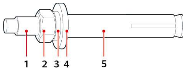
Figura 4-14 Partes de un tornillo de expansión
