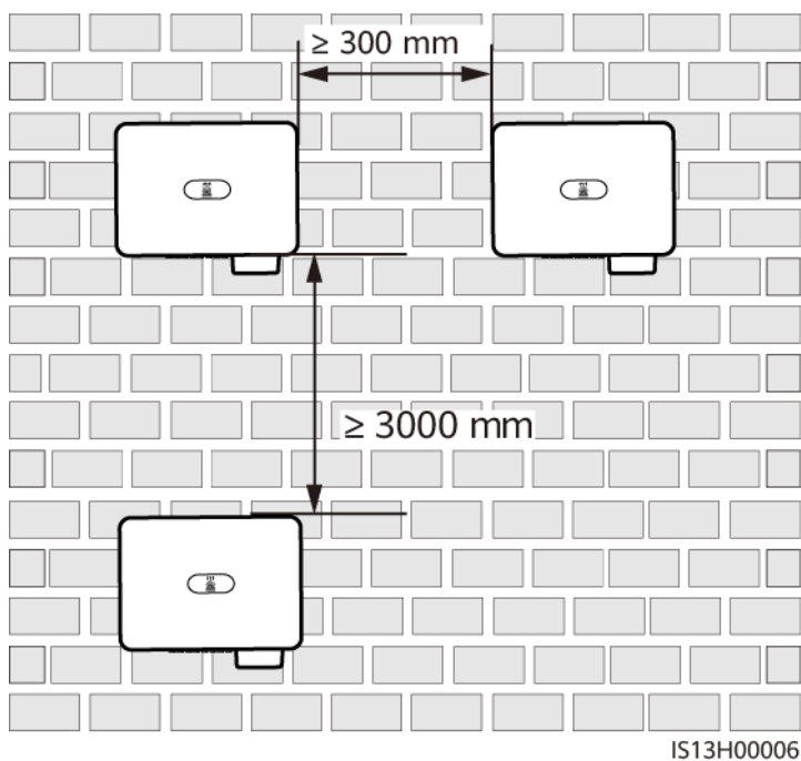
Figura 4-6 Instalación espaciada de doble fila en pared (no recomendada)
