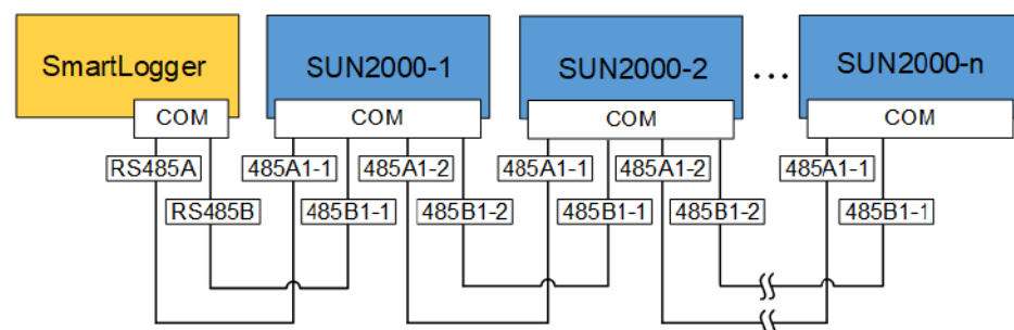
Figura 5-21 Conexión en red del SmartLogger
