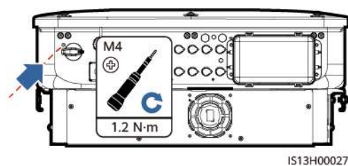
Figura 4-16 Instalación del tornillo de fijación correspondiente al interruptor de CC
