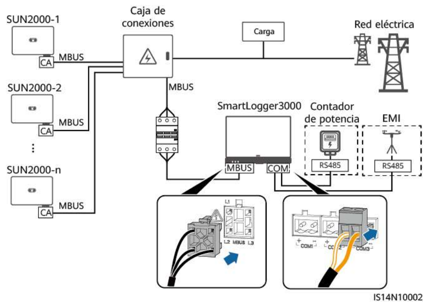
Figura 5-23 Comunicación MBUS (situaciones de suministro comercial e industrial en China)
