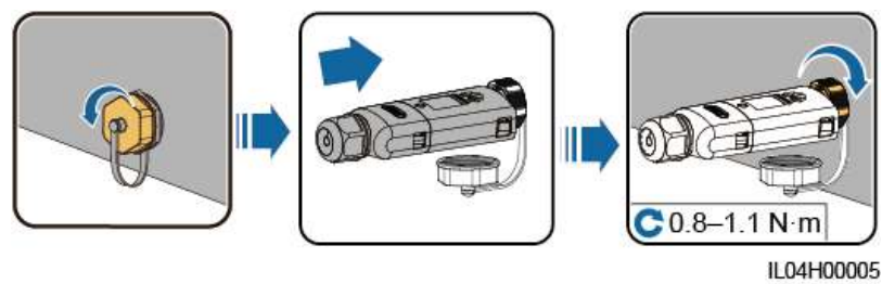
Figura 5-16 Instalación del Smart Dongle WLAN-FE (comunicación WLAN)
