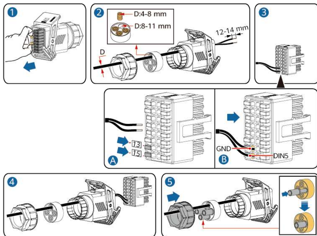
Figura 5-30 Conexión del cable
