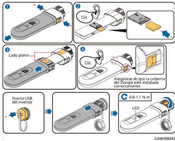
Figura 5-15 Instalación del Smart Dongle 4G (SDongleB-06)
