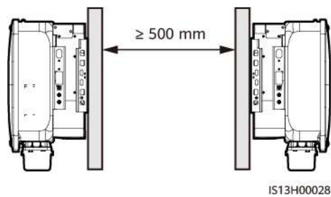
Figura 4-9 Instalación espalda con espalda de doble fila en soporte (no recomendada)
