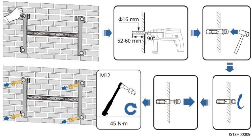
Figura 4-15 Instalación de los tornillos de expansión
