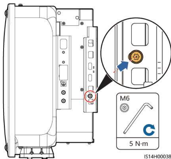
Figura 4-18 Ajuste de la tuerca
