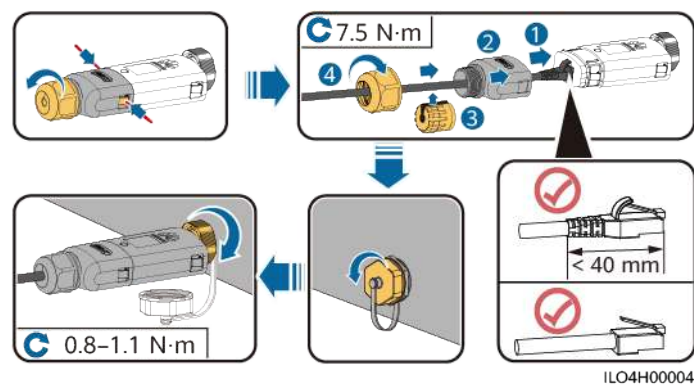
Figura 5-17 Instalación del Smart Dongle WLAN-FE (comunicación FE)
