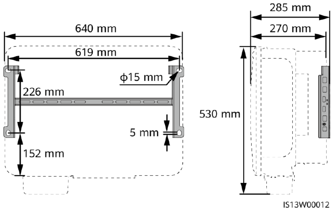
Figura 4-12 Dimensiones de la ménsula de montaje
