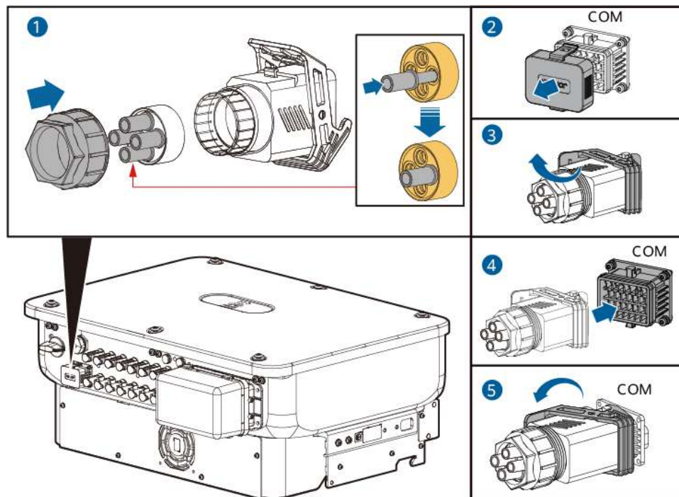
Figura 5-19 Fijación del conector del cable de señal
