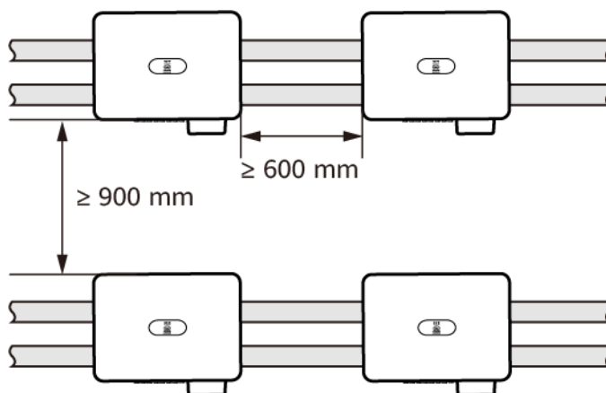
Figura 4-7 Instalación espaciada de doble fila en soporte (recomendada)
