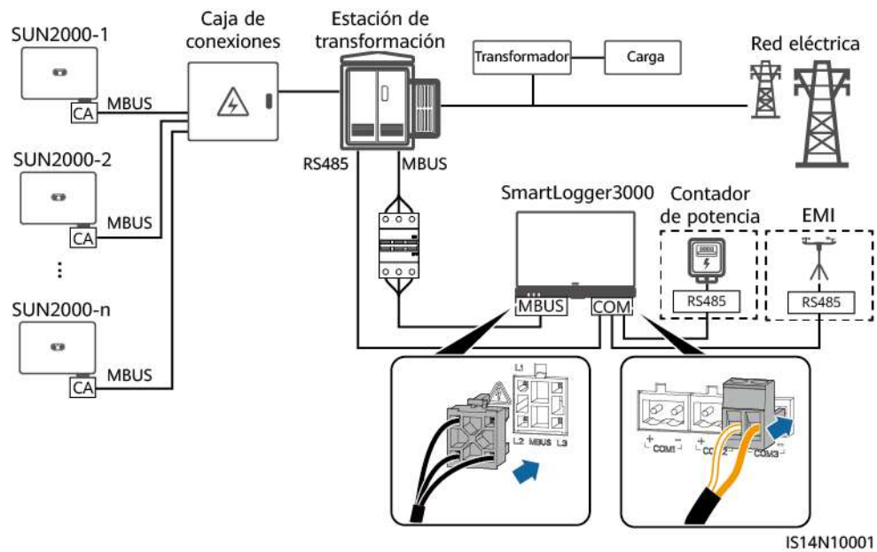
Figura 5-22 Comunicación MBUS (situaciones de suministro a gran escala)
