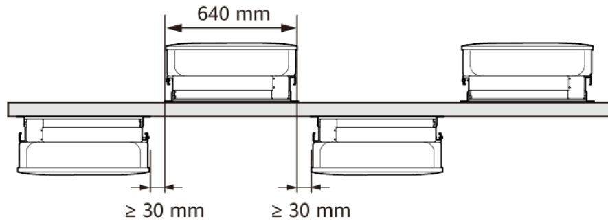
Figura 4-8 Instalación de dos lados de una sola fila en soporte (recomendada)
