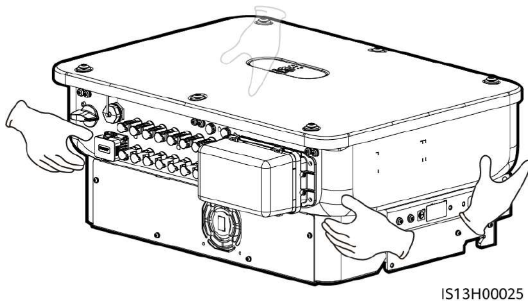
Figura 4-10 Traslado del SUN2000
