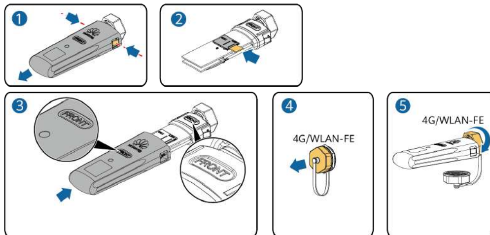
Figura 5-14 Instalación del Smart Dongle 4G (SDongleA-03)
