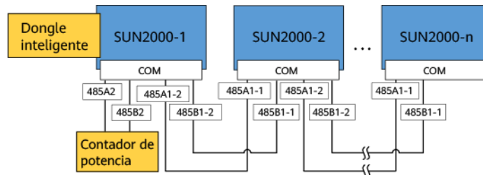
Figura 5-20 Conexión en red del Smart Dongle
