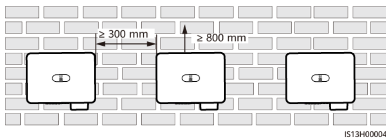
Figura 4-3 Instalación horizontal (recomendada)
